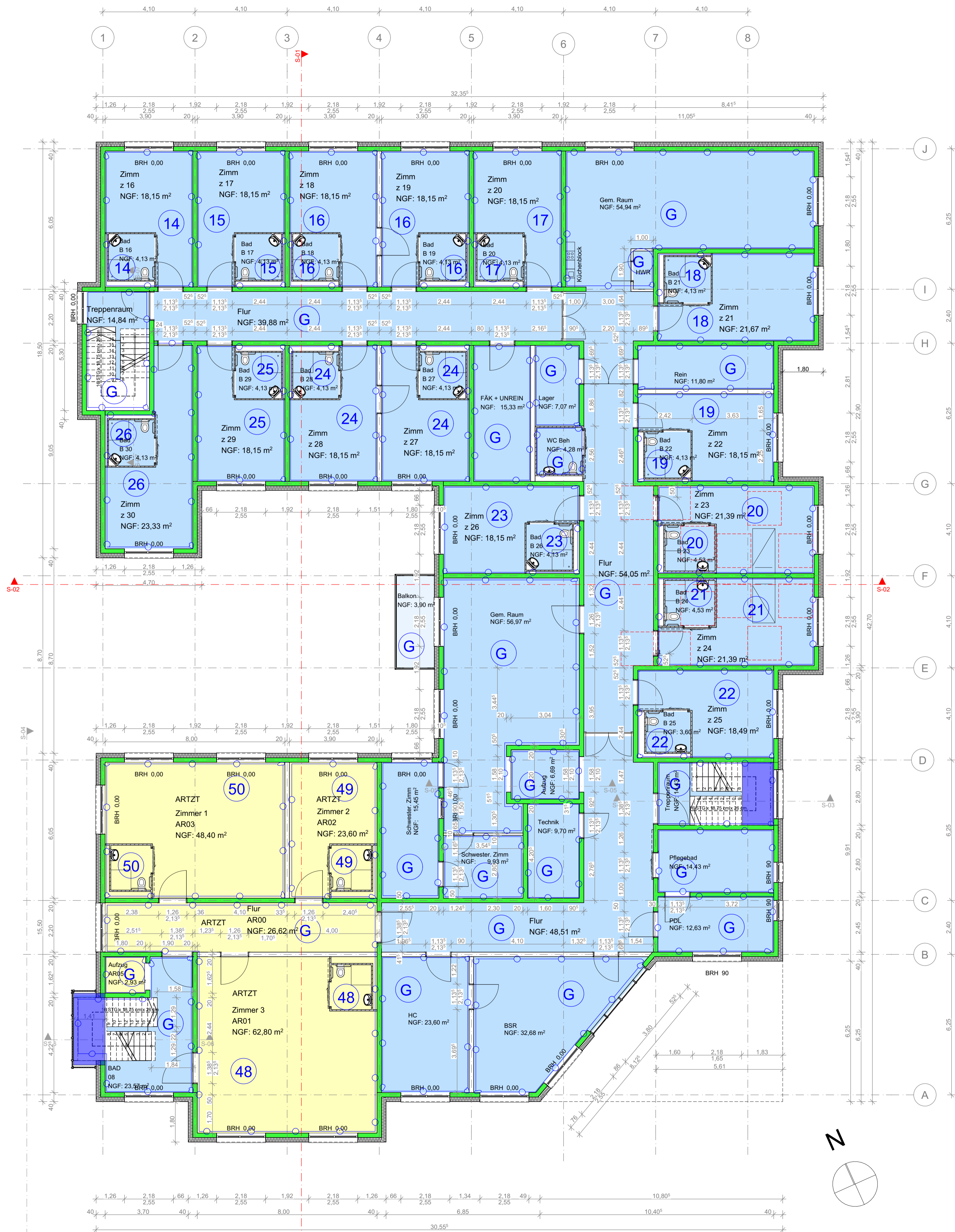
1. OBERGESCHOSS BGF: 1148 M2
